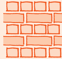
イギリス積み
